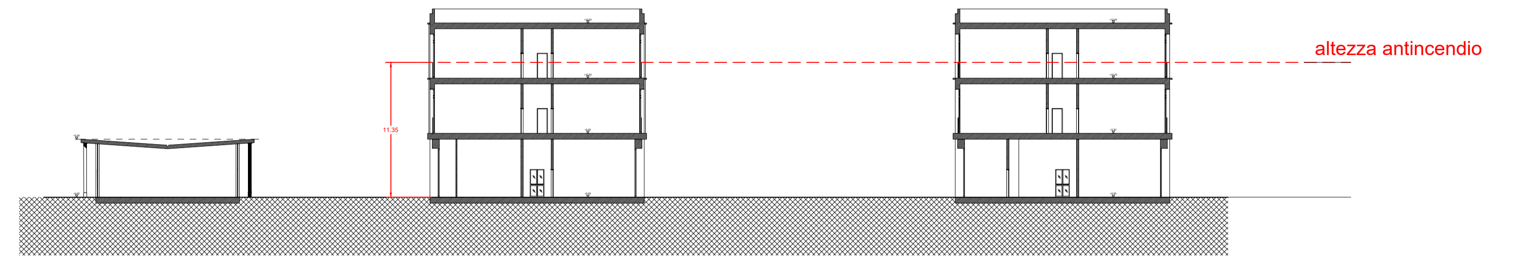
SEZIONE AA (con indicazione altezza antincendio)
