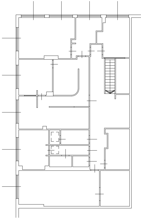
PIANTA PIANO PRIMO 1:200 Situazione Sovrapposto
