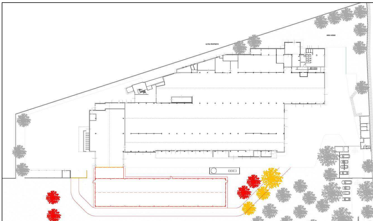
Figura 7: planimetria dell'area dell'area di intervento (in rosso l'ampliamento previsto)
