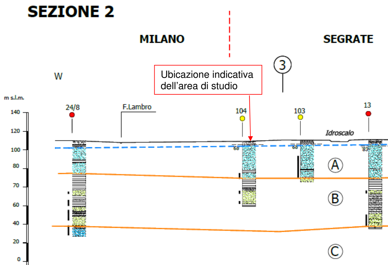
Fig. 7a – Sezione 2 di riferimento
