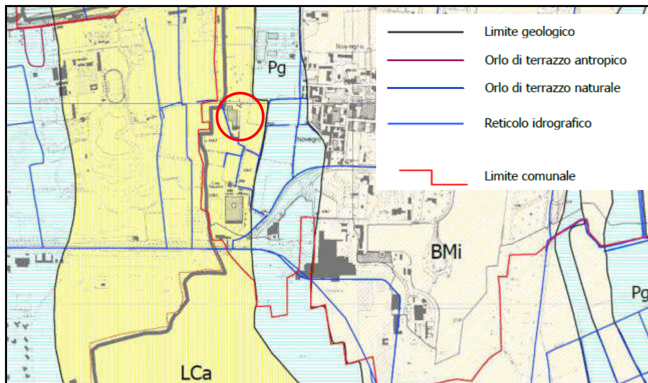
Fig. 5 – Inquadrimento geomorfologico e geologico (estratto dal PGT comunale)
