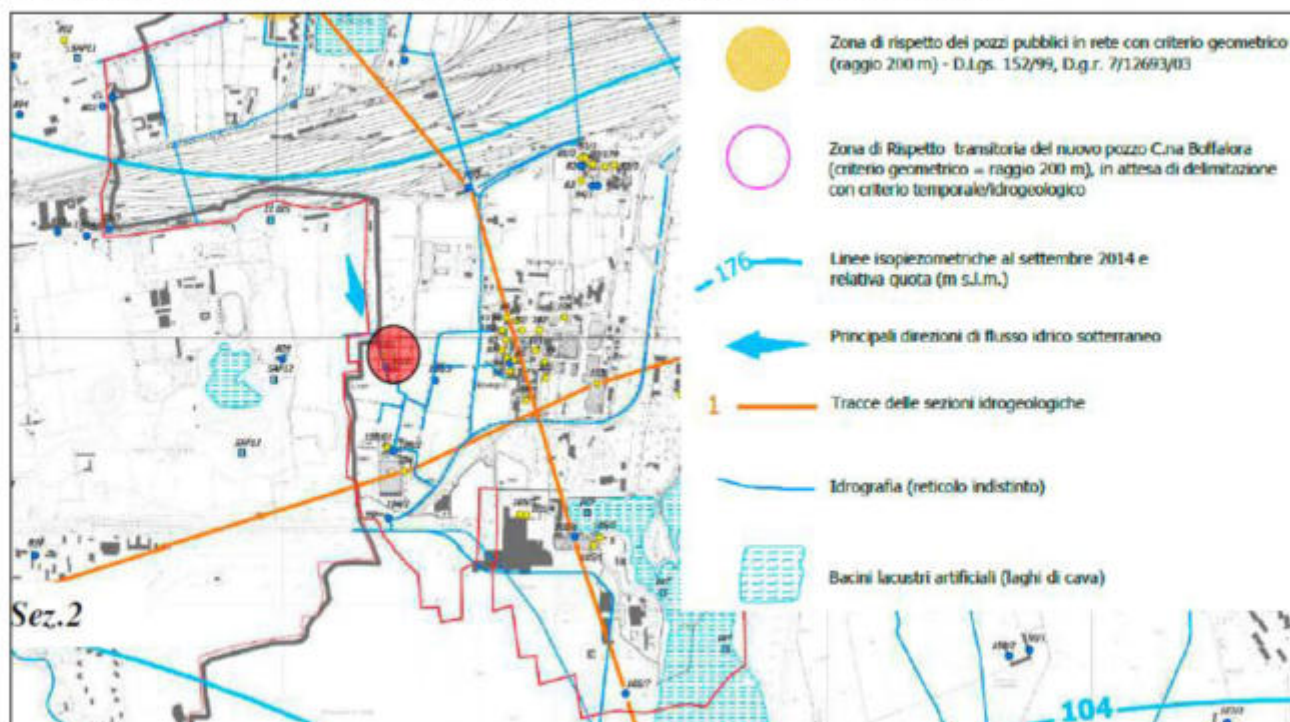
Figura 8: Stralcio Tavola GEO 02 "Caratteri idrogeologici"
