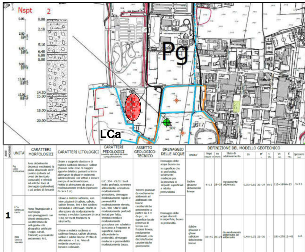
Fig. 9 – Caratteristiche geologico-tecniche (estratto dal PGT comunale)
