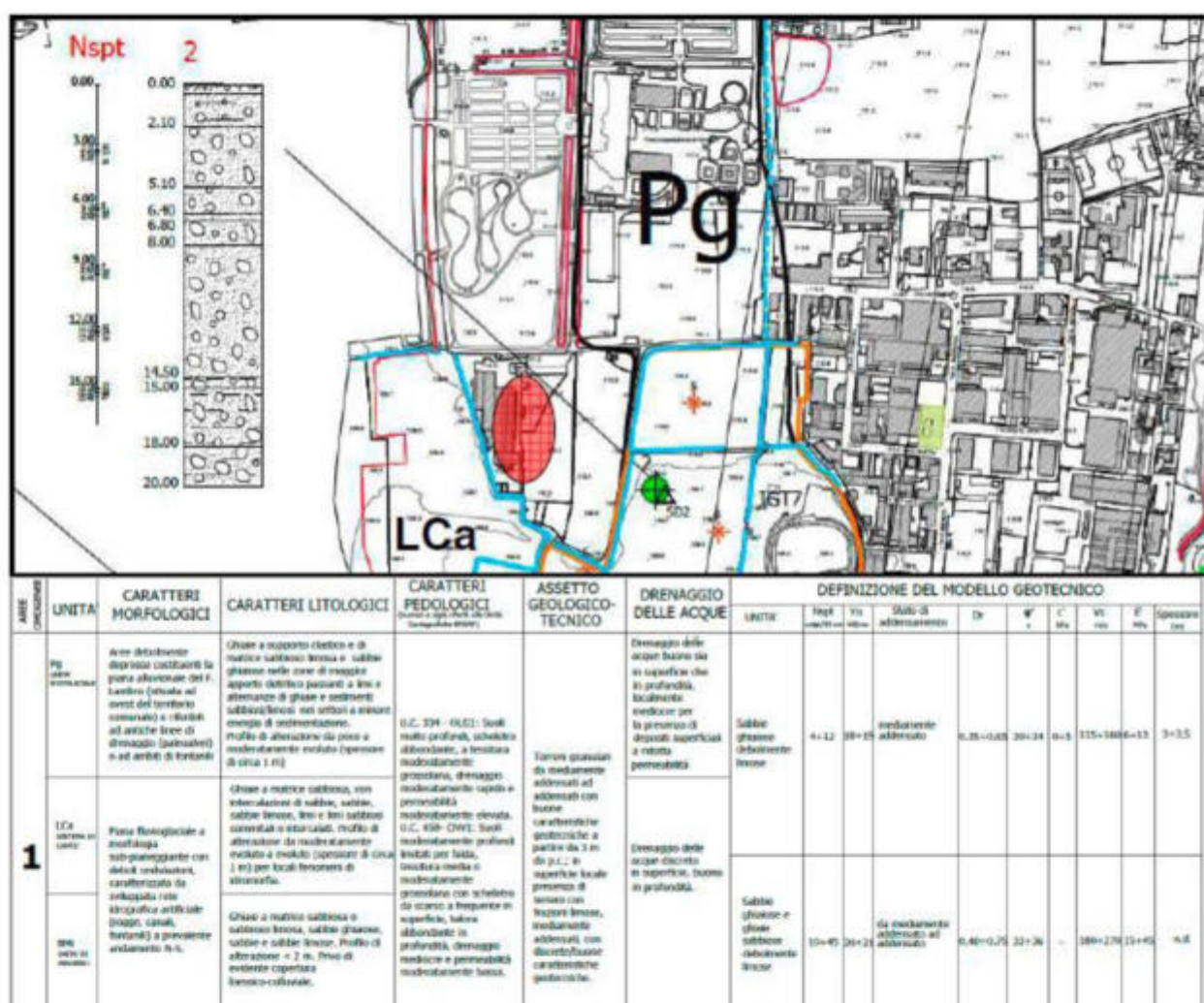
Figura 11: Stralcio Tavola GEO 05 (Fonte: Componente Geologica del PGT di Segrate)
