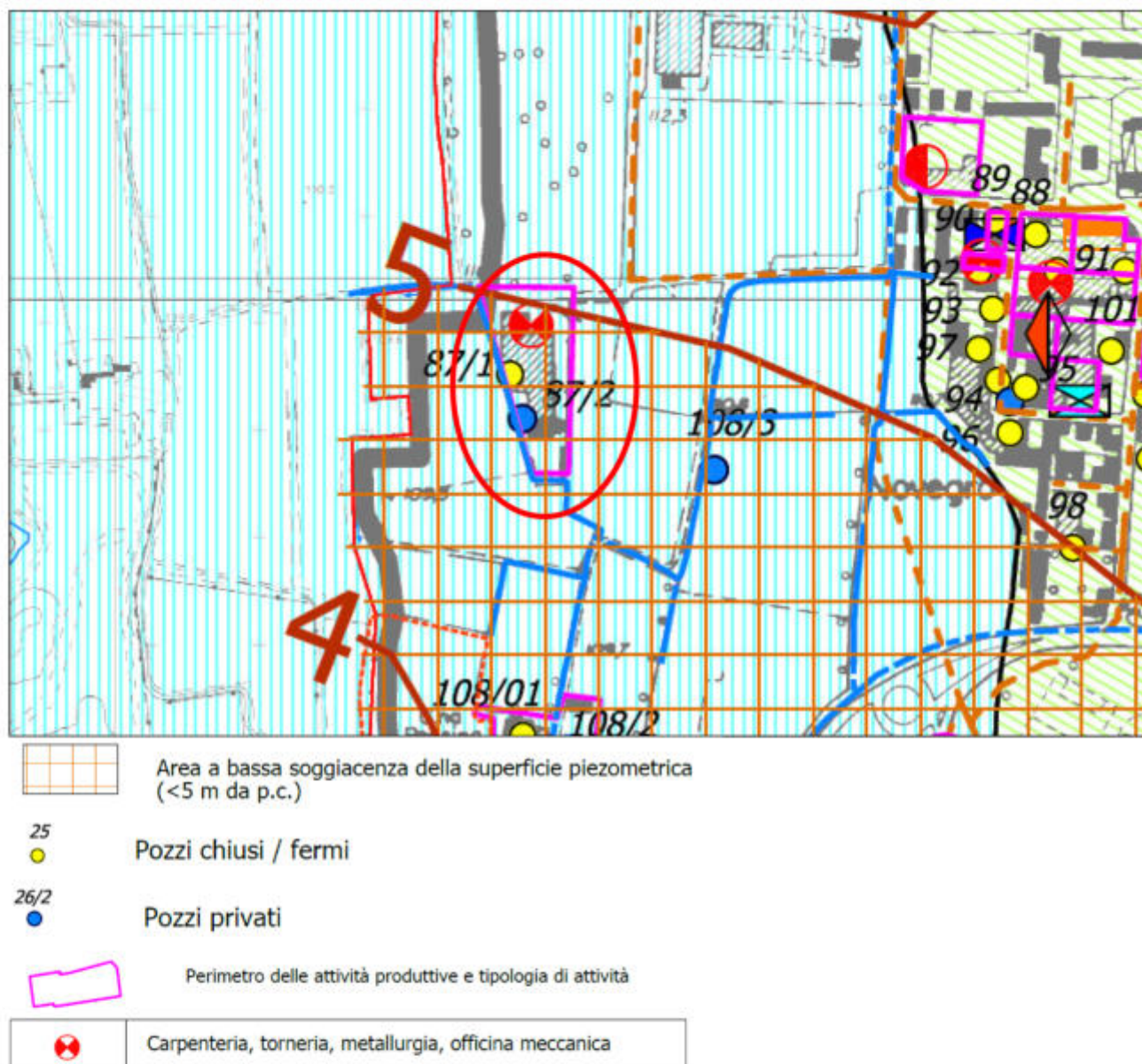
Figura 10: Stralcio Tavola GEO 04 (Fonte: Componente Geologica del PGT di Segrate)
