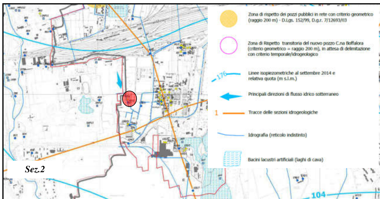
Fig. 7 – Inquadramento idro-geologico (estratto dal PGT comunale)
