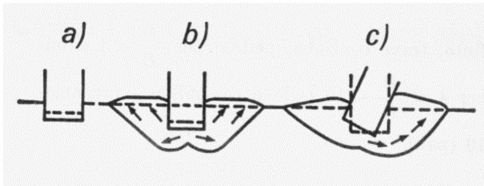
Fig. 23 - Comportamento del terreno sotto una fondazione, sulla quale il carico aumenta progressivamente fino a produrre la rottura. (a) fase pseudo-plastica – cedimento minimo (b) fase plastica – cedimento, rottura per taglio del terreno e rigonfiamento laterale (c) fase di rottura – lesioni e/o crolli della struttura superficiale.
