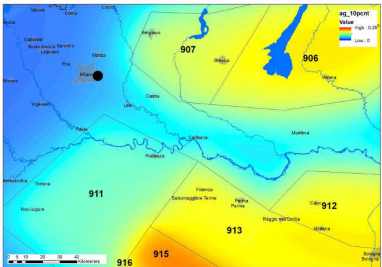
Figura 16: Zonazione sismogenetica ZS9: l'Italia del Nord (da Meletti C. & Valensise G., 2004).
