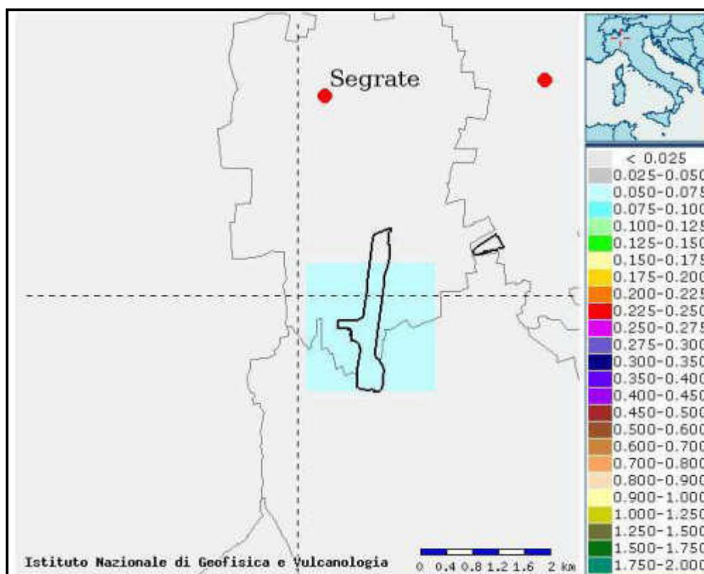
Figura 17: Mappatura dell’accelerazione orizzontale massima del terreno ( a_g ) con tempi di ritorno di 475 anni.
