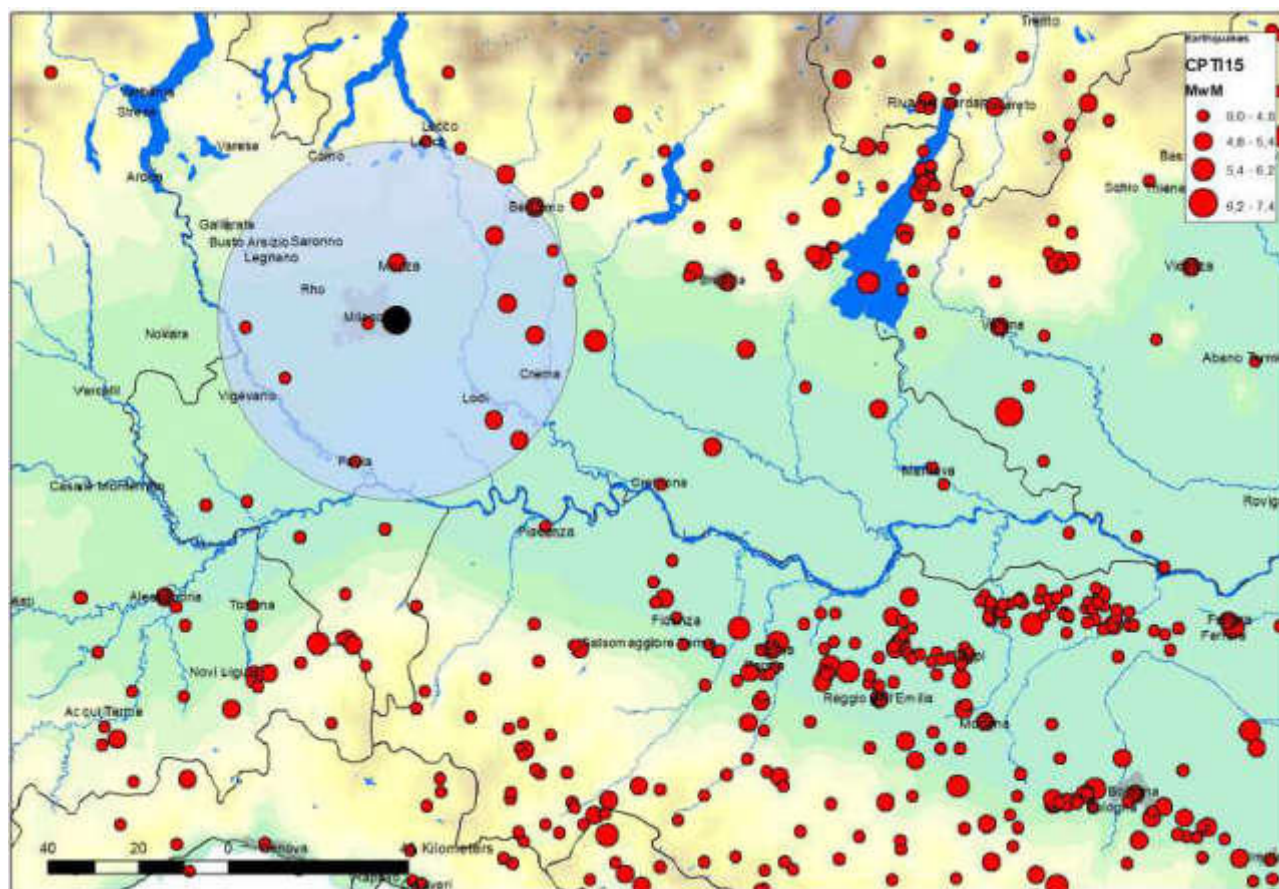
Figura 14: Distribuzione degli eventi sismici estratta dal catalogo parametrico dei terremoti italiani del 2015 (CPTI 15) che mostra gli epicentri dei terremoti più significativi avvenuti nell'area interessata e zone limitrofe.
