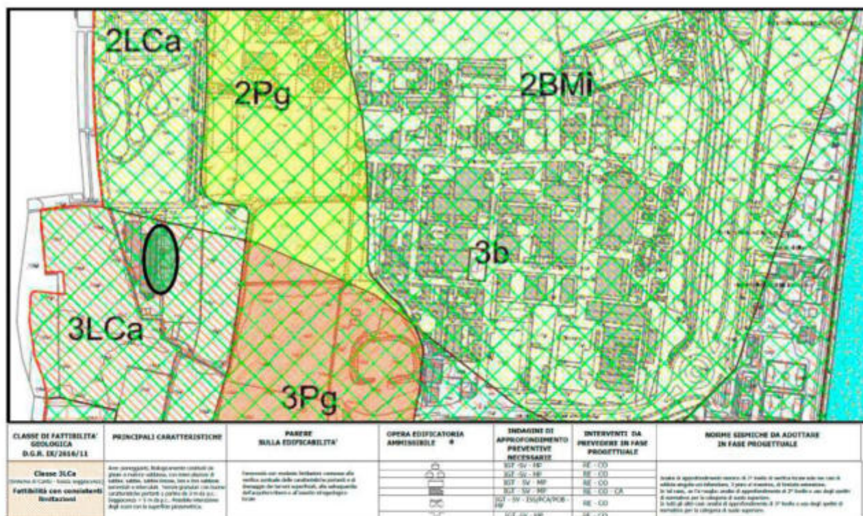
Figura 16: Stralcio Tavola GEO 09 (Fonte: Componente Geologica del PGT di Segrate)
