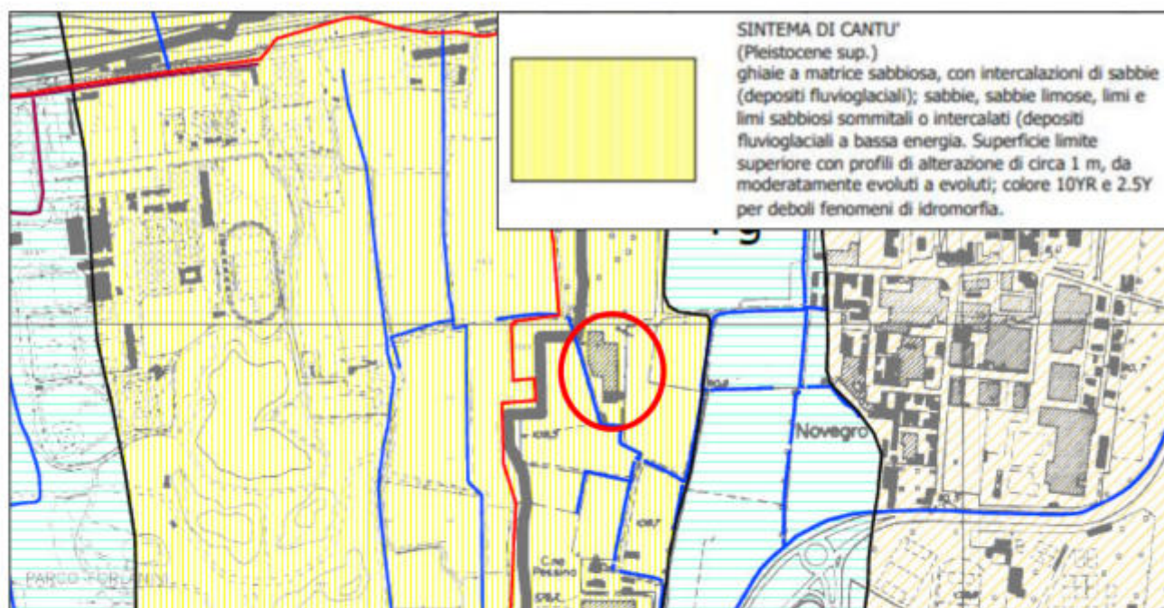
Figura 7: Stralcio Tavola GEO 01 "Caratteri geologici e geomorfologici"
