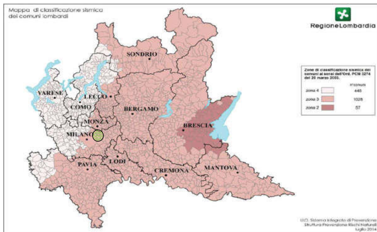
Figura 20: Classificazione sismica vigente dei Comuni della Regione Lombardia
